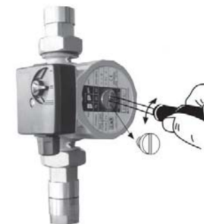
Desbloquear eje
