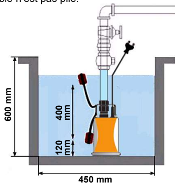
Dimensions minimales
