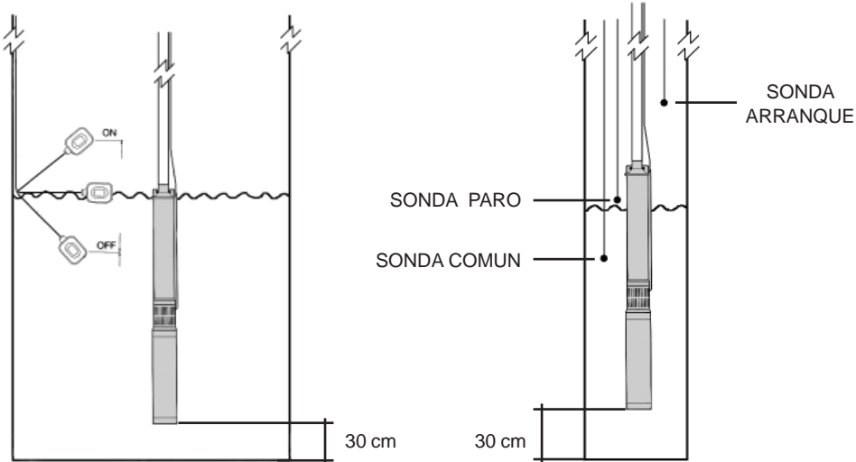
Instalación en pozo abierto
