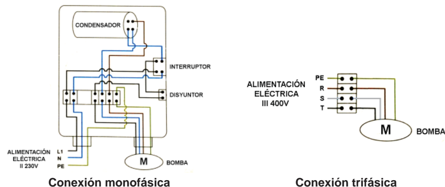
Conexión monofásica
